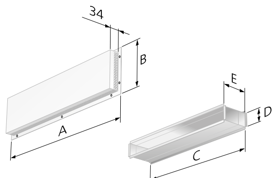
Abb. 2. ROT, Abmessungen.
