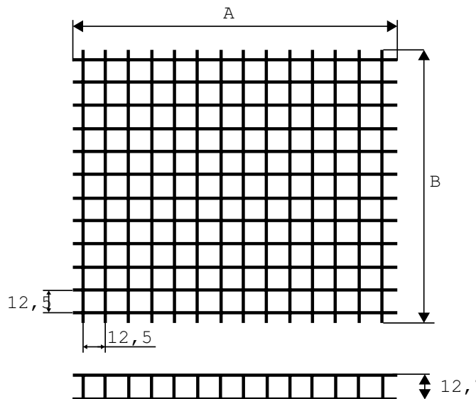
Figur 3. Mått RASTER (mm).
