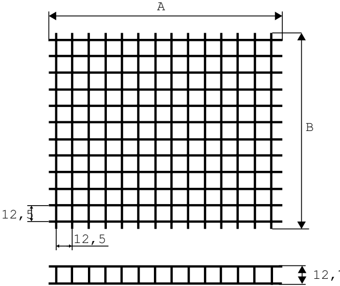
Kuva 3. RASTER mitat (mm).
