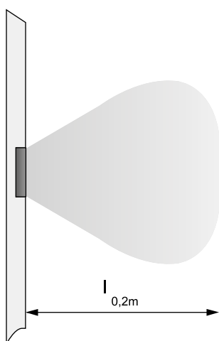
Figur 5. Isovel. Spridningsbild standard 0°.
