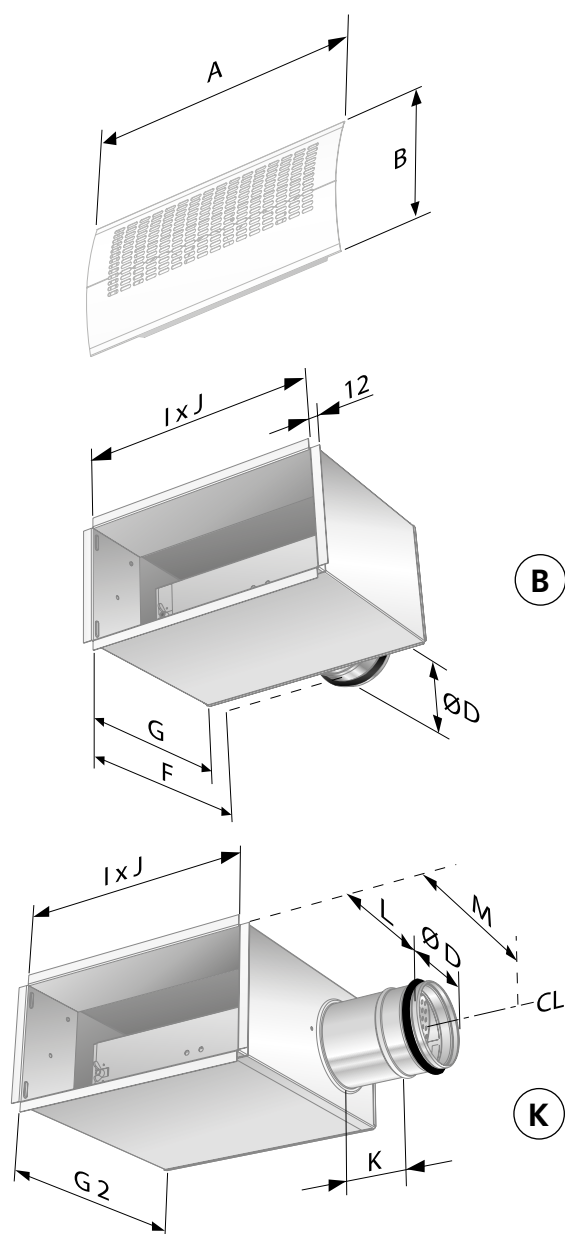
Figur 7. PELICAN W + ALV.
