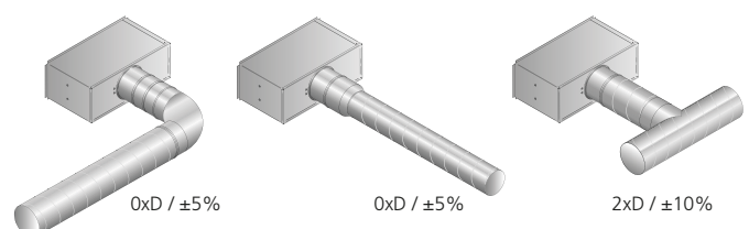
Figur 2. Monteringsalternativ, gäller för alla anslutningar (B, K)
