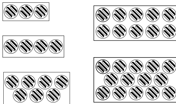
Figur 4. Luftriktariinställning för alternativ spridningsbild 45° till vänster.
