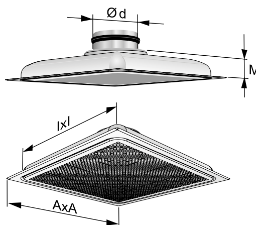
Abbildung 4. PELICAN CE HF.
