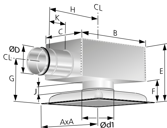
Abbildung 5. PELICAN CE HF mit ALS
