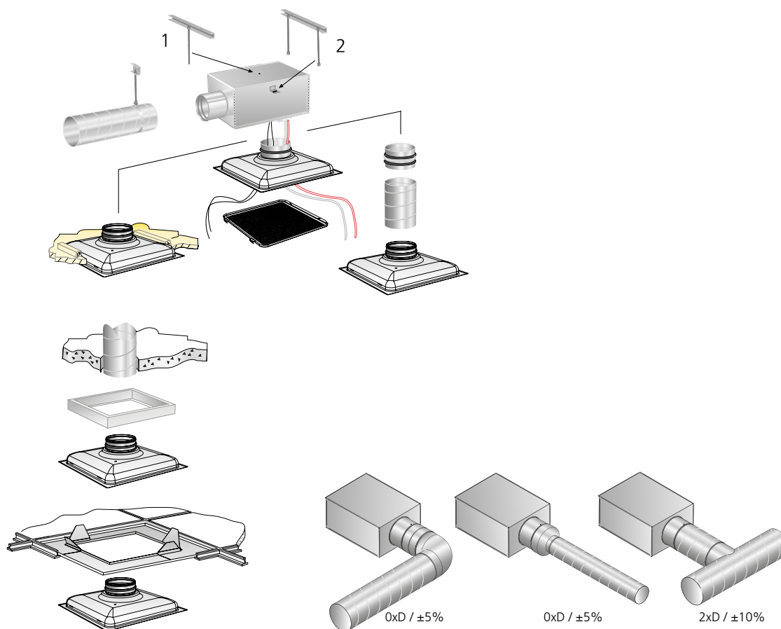
Abbildung 2. Montagealternativen.
