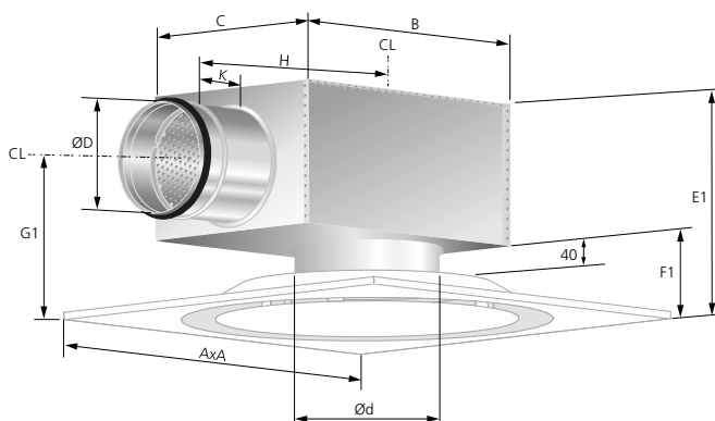
Figur 13. KITE CC med anslutningslåda ALS eller REACT ALS. CL = Centrumlinje.
