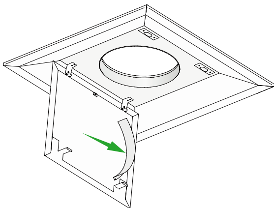
Figur 6. Alternativ 1, montering av avskärmning i spridardel.
