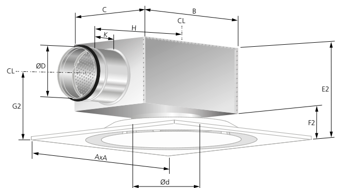
Figur 14. KITE CC med anslutningslåda ALS. Låg bygghöjd.
