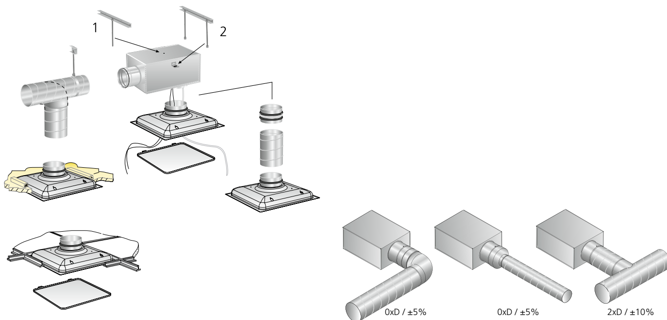
Figur 3. Monteringsalternativ för anslutningslåda ALS. Se REACT ALS produktblad för monteringsalternativ med aktiv anslutningslåda.
