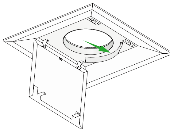
Figur 7. Alternativ 2, montering av avskärmning i mellanlåda.
