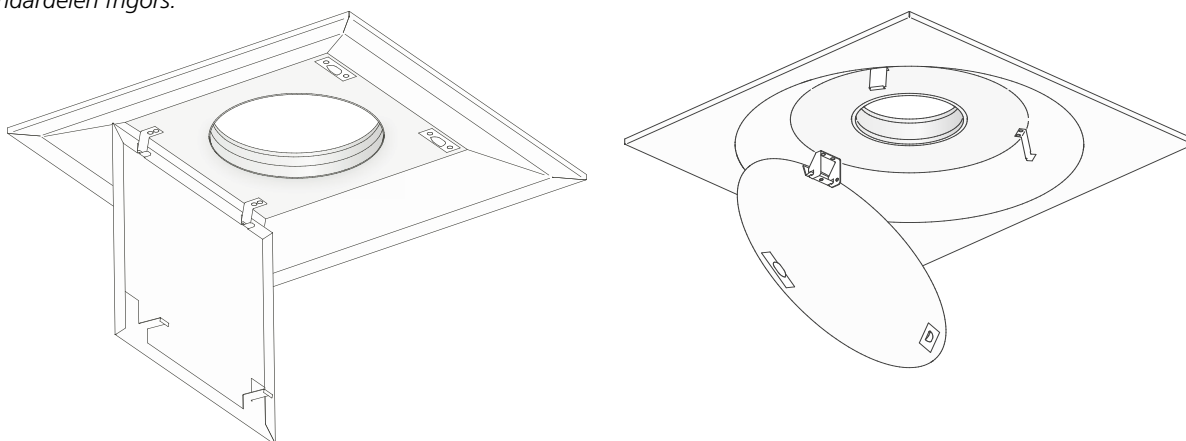
Figur 2. Easy Access, demontering av spridardel.
