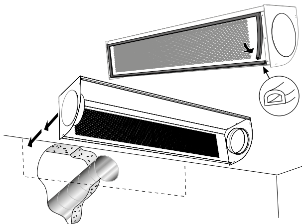
Figur 2a. IBIS W, bakanslutning. Applicering av tätningslist.
