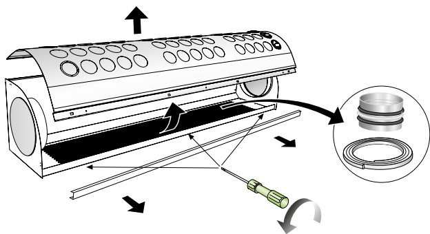
Figur 1. IBIS W, Demontering av frontplåt.
