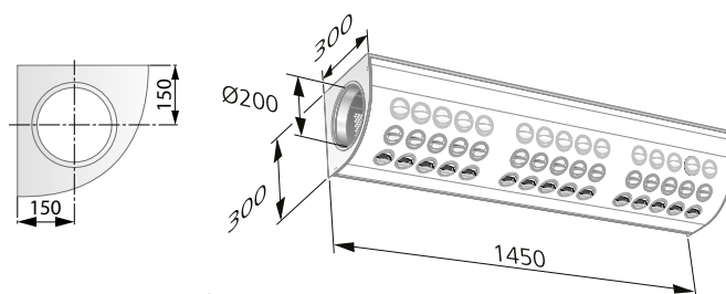
Figur 5. IBIS W mått.
