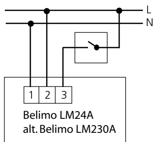
Kuva 1. FALCON HF:n kytkentäkaavio, moottorinohjaus 2-pistesäädöllä. Vaihtokytkin ei sisälly toimitukseen.
