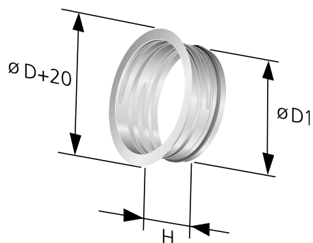
Figur 5. Monteringsramme EXCT 2.
