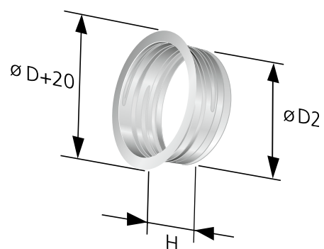
Figur 6. Monteringsramme EXCT 3 Monteringsramme til tilslutning direkte mod kanaldel med nippel, f.eks. en kanalbøjning.
