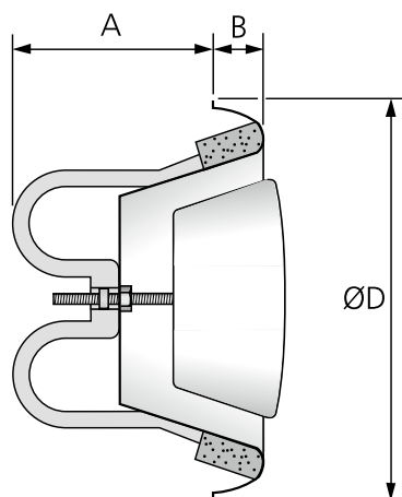
Figur 4. Fraluftarmatur EXC.
