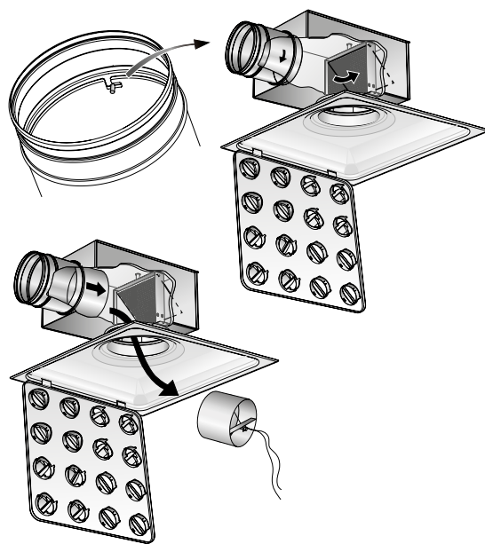
Kuva 4. Pellin irrotus.
