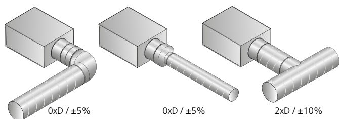
Figur 3. Monteringsalternativ.
