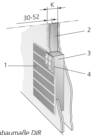
Abbildung 4. Einbaumaße DIR
