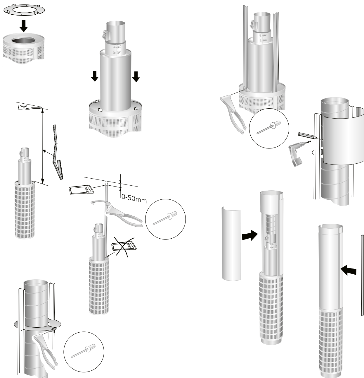
Figur 3. Montering kanalinklädnad.
