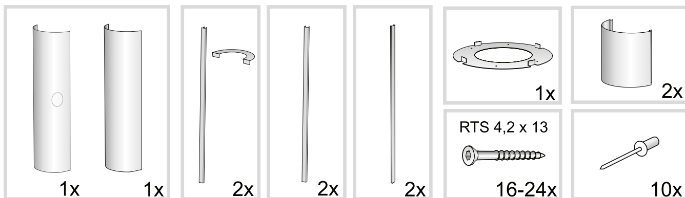
Figur 2. Översikt ingående delar.
