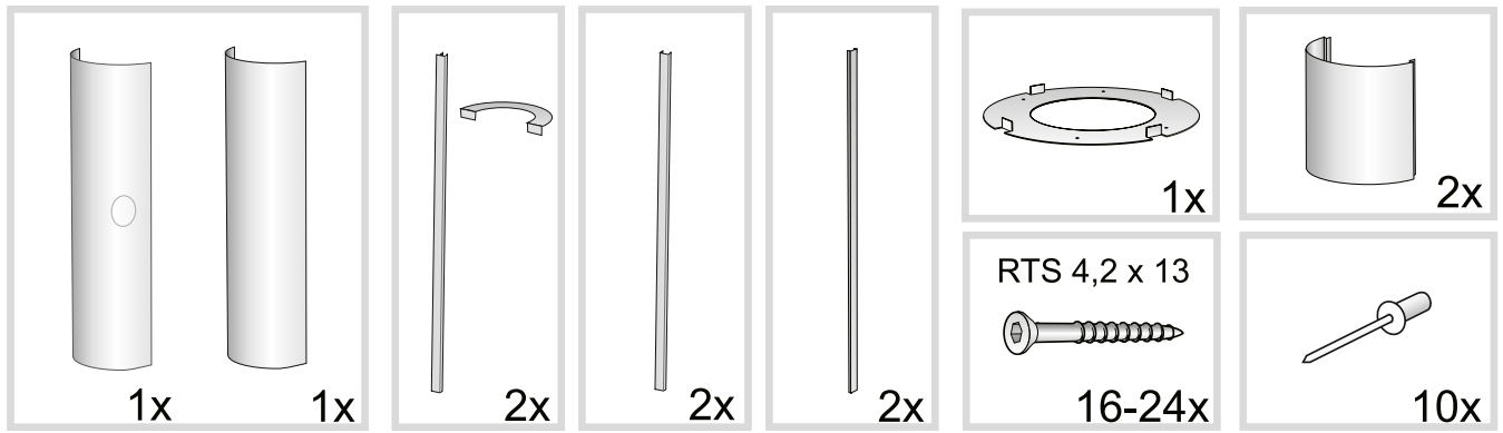
Kuva 2. Sisältyvät osat.
