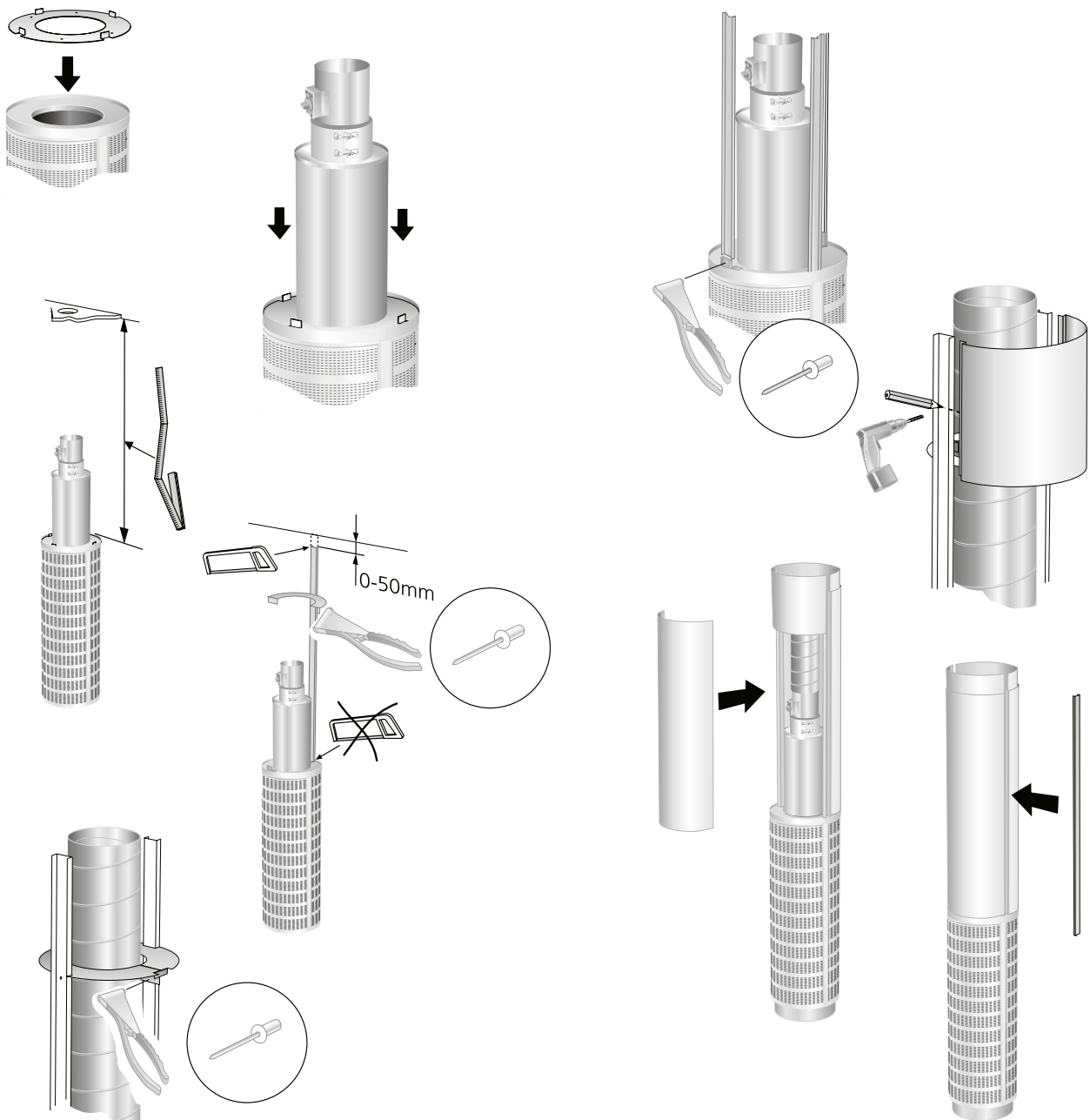
Kuva 3. Asennus, kanavaverhoilu.
