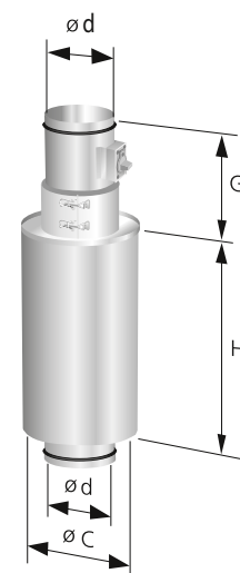
Kuva 7. DCP varustettuna kanavaverhouksella ja sokkelilla. 1. Koko 125-315: 2400-2750. Koko 400, 500, 630: 2850-3200. Muita pituuksia tilattaessa on aina ilmoitettava huoneen kokonaiskorkeus.
