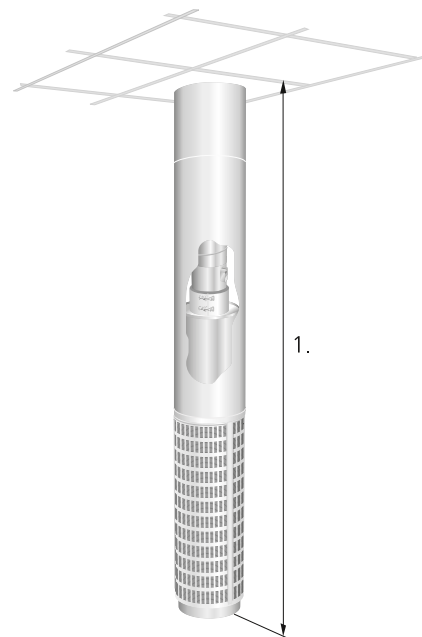
Kuva 7. DCP varustettuna kanavaverhouksella ja sokkelilla. 1. Koko 125-315: 2400-2750. Koko 400, 500, 630: 2850-3200. Muita pituuksia tilattaessa on aina ilmoitettava huoneen kokonaiskorkeus.
