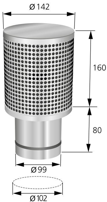
Kuva 4. DCC. Mittausyksikkö = mm. Paino: 1,2 kg. Aukontekomitta = Ø102 mm.
