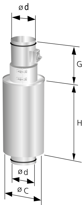
Figur 4. Reguleringsenhed REG.
