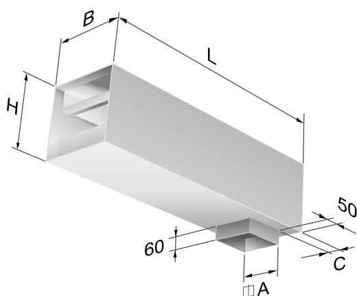
Figur 4. Mått CTK.
