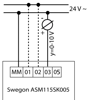
Kuva 4. Moottorilla varustetun CKD 2 kytkentäkaavio. Moottori 0-10V säädöllä. Potentiometri ei sisälly toimitukseen.
