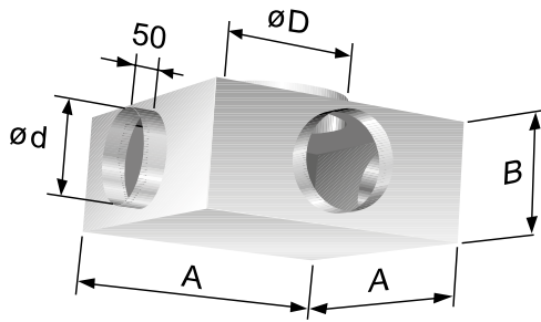
Kuva 9. CKDT 1, 4 hajottimien, 0° pystykulma.
