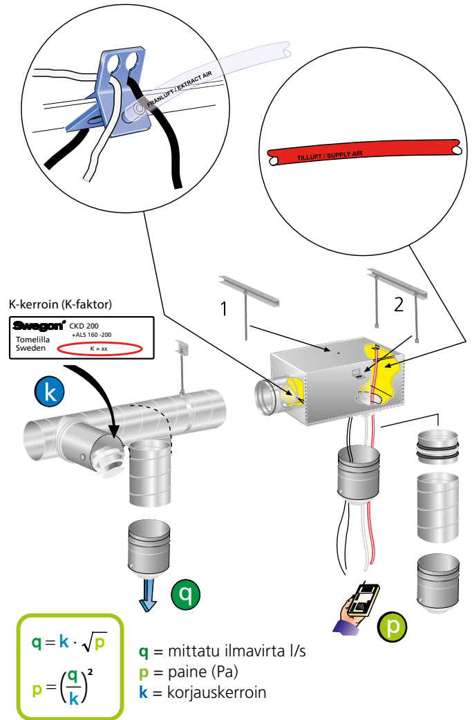
Kuva 1. Asennus, säätö.
