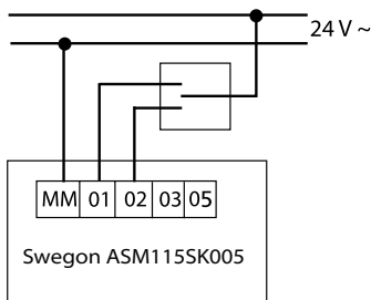
Kuva 3. Moottorilla varustetun CKD 2 kytkentäkaavio. Moottori 3-pisteohjauksella. Vaihtokytkin ei sisälly toimitukseen.
