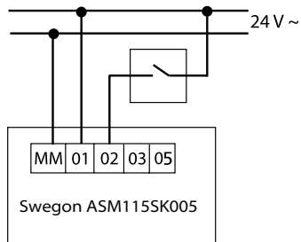
Kuva 2. Moottorilla varustetun CKD 2 kytkentäkaavio. Moottori 2-pisteohjauksella. Vaihtokytkin ei sisälly toimitukseen.
