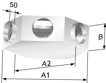
Kuva 10. CKDT 1, 6 hajottimien, 0° pystykulma.
