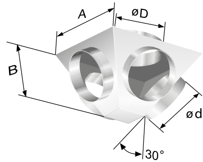
Kuva 11. CKDT 1, 4 hajottimien, 30° pystykulma.
