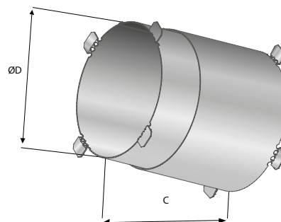
Abb. 5. VGC, Abmessungen.
