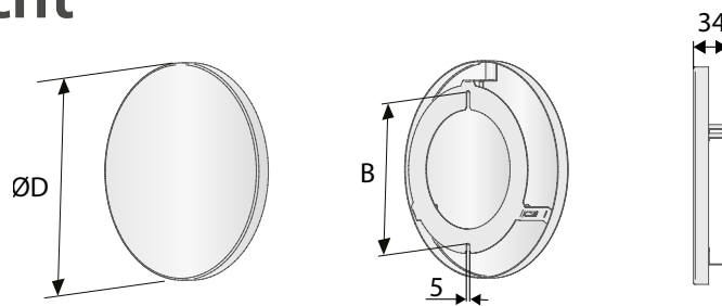
Abb. 4. CIRCO, Abmessungen.
