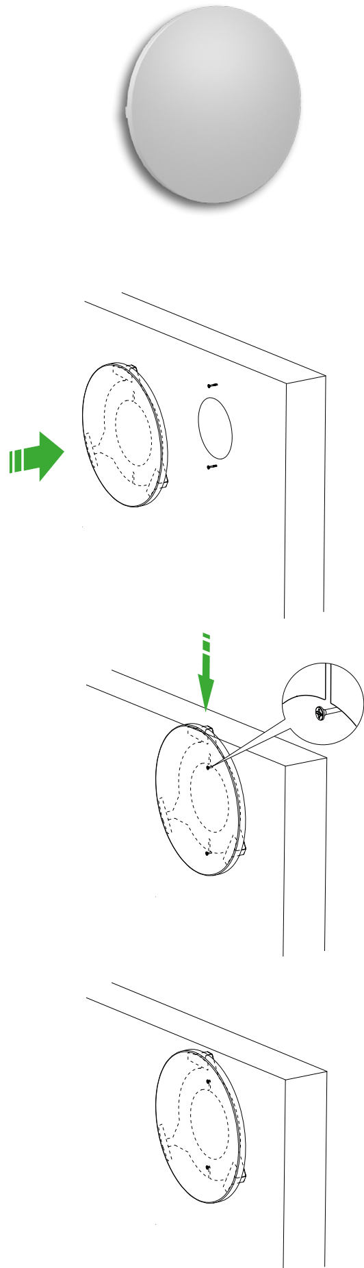
Abb. 1. Montage
