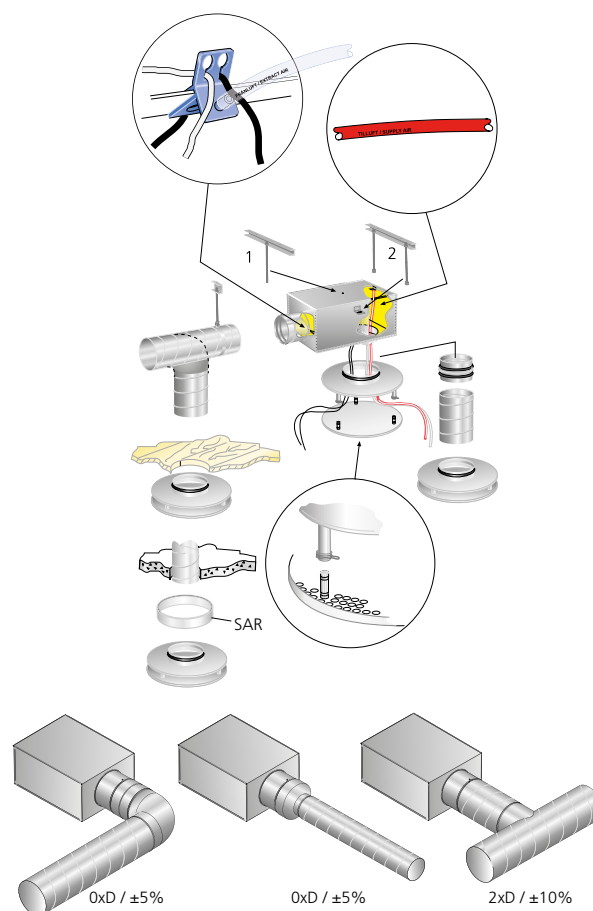
Abbildung 1. Montage. Einregulierung.
