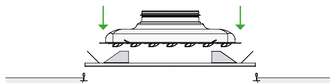
Figur 1. Montering av ADAPTER och luftdon 500.
