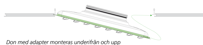
Figur 2. Montering av ADAPTER och luftdon 600.
