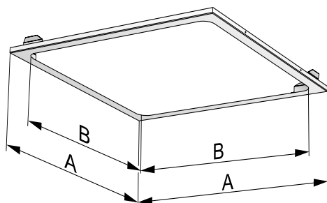
Figur 3. ADAPTER kvadratisk luftdon.
