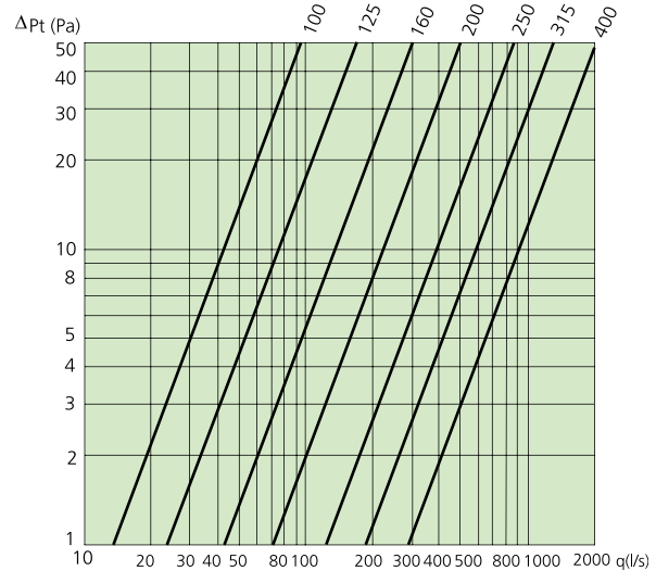
Käyrästä 1. Ilmavirta – painehäviö, SORDO-C 100- 400
