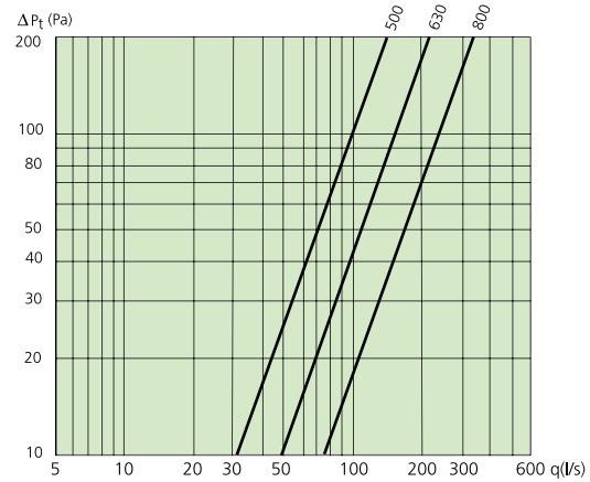
Käyrästä 2. Ilmavirta – painehäviö, SORDO-C 500- 800
