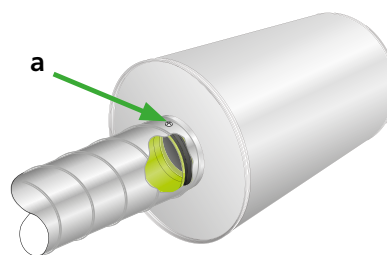
Kuva 1. Paloturvallisuuden vuoksi kanavat kiinnitetään liittimen sisään valettuun peltireunaan ruuvilla tai popniitillä (a).
