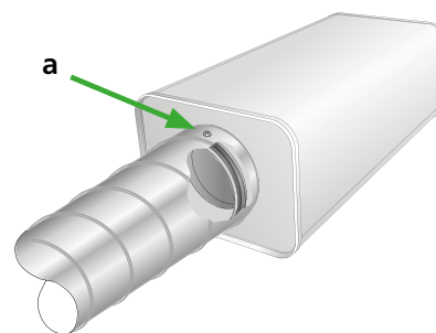
Figur 1. Av hensyn til brann sikkerheten er tilkoblingskanalen festet til platekanten som er festet inne i tilkoblingsboksen med en skrue eller popnagle (a).
