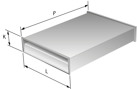
Kuva 3. MORENDO – mittapiirustus.
