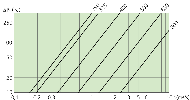
Schéma 1. Perte de charge – Débit d'air, CLA-B
