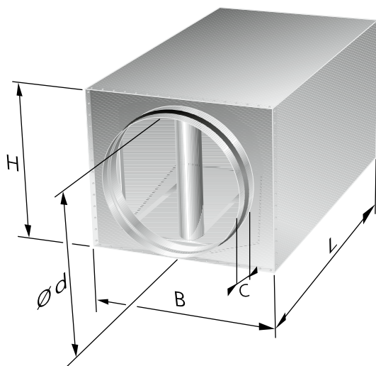
Kuva 3. CLA-B – mittapiirros
