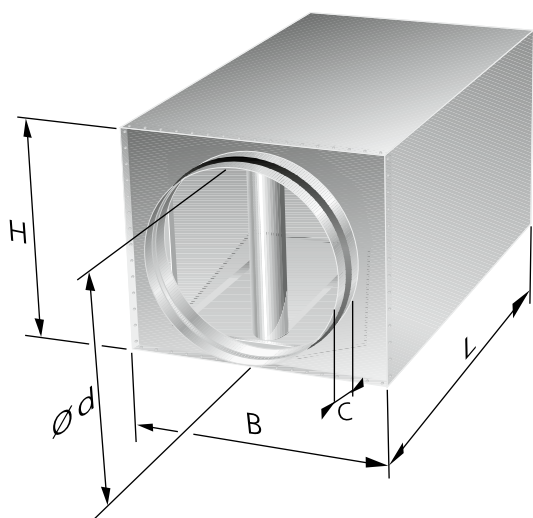
Figur 3 CLA-B – målskitse
