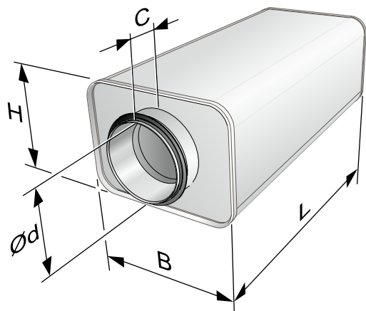
Figur 2. CLA-A – måttskiss
