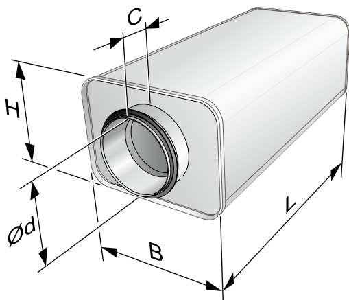
Abb. 2. CLA-A – Maßskizze
