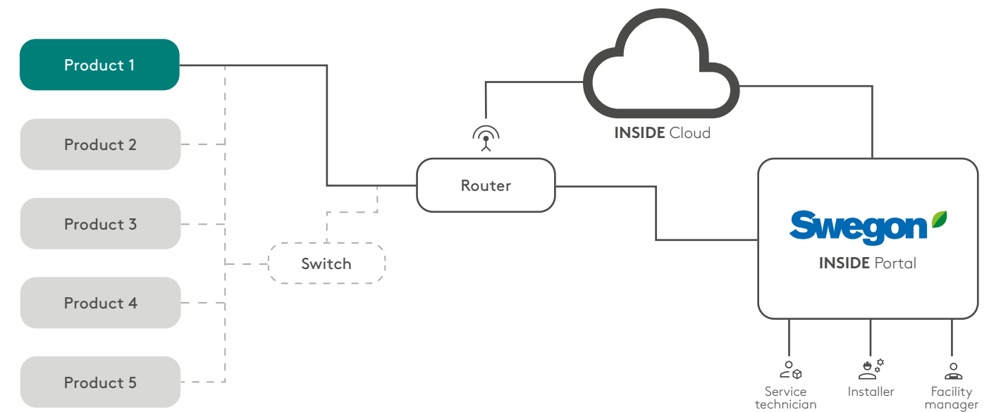
Figur 5. Systemöversikt och anslutningar.
