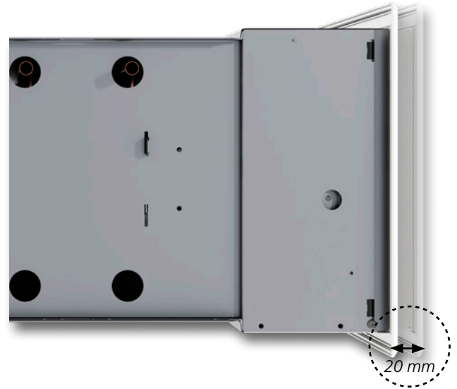
Kuva 3. Tulo- ja poistoilmasäleikön säätö.
