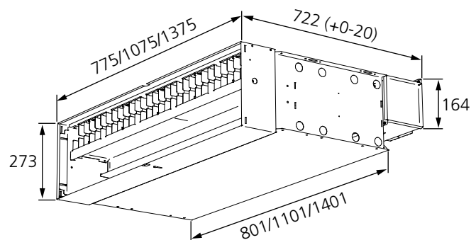
Kuva 17. Mitat ilman säleikköä.
