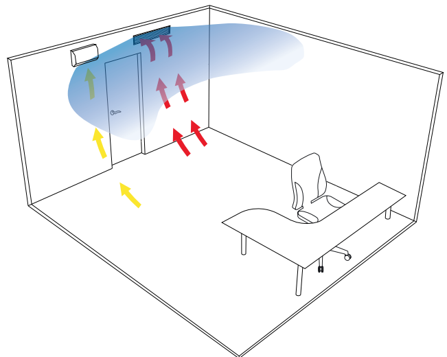
Kuva 10. Ilmanjako REACT Paragon Wall -tuotteella yksittäisessä toimistossa.
