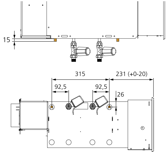
Kuva 14. Mitat, ripustus.
