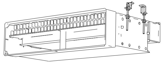
Kuva 12. REACT Paragon Wallin asennus, tässä ripustettu käyttäen kierretankoja.
