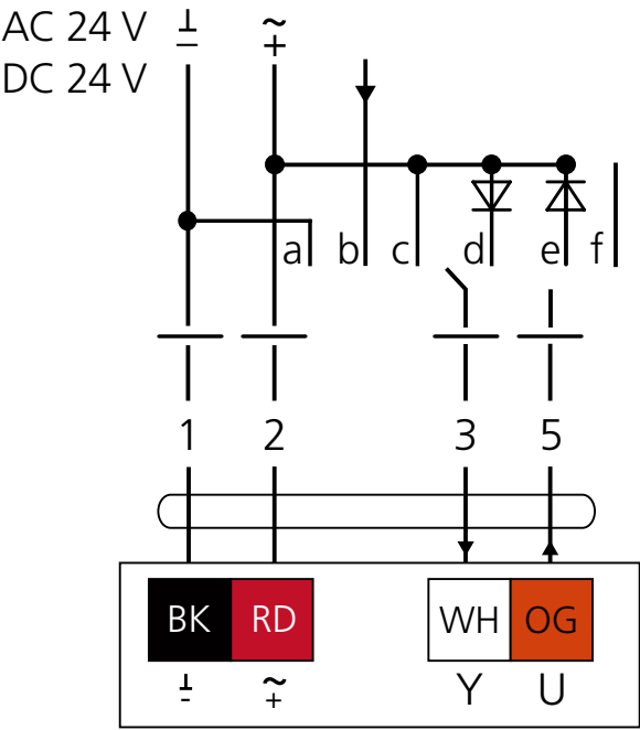
Abb. 9. Schaltplan.
