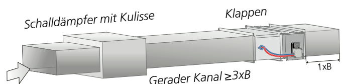
Abb. 8. Anforderungen an gerade Strecken 3 x B bei Schalldämpfern mit Kulissee. Gilt sowohl für Zu- als auch Abluft.
