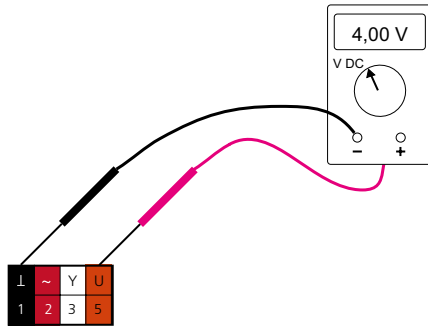
Abb. 16. Zeigt den Anschluss des Voltmeters für die Kontrolle des Istwerts.
