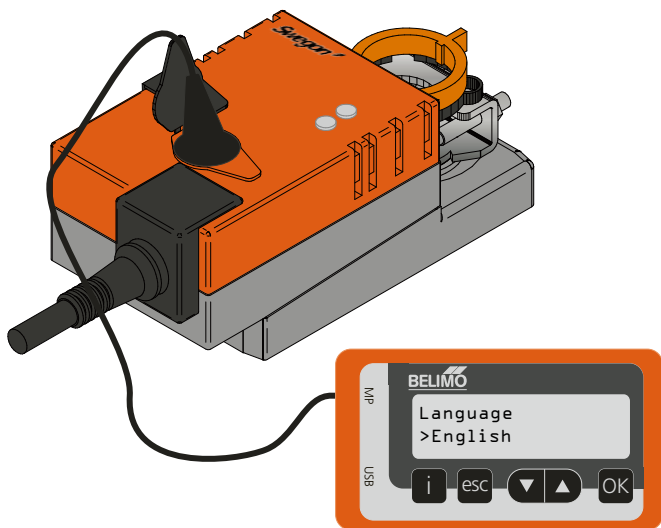
Abb. 15. Belimo ZTH EU – Handterminal zur Einstellung und Ablesung der Parameter des Stellantriebs.
