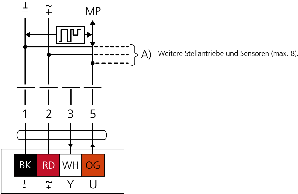
Abb. 10. Schaltplan MP-Bus.
