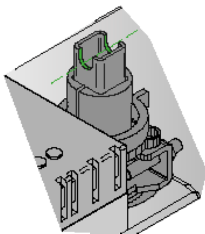
Abb. 18. Der Ausschnitt in der Klappenwelle zeigt die Stellung der Klappe an.
