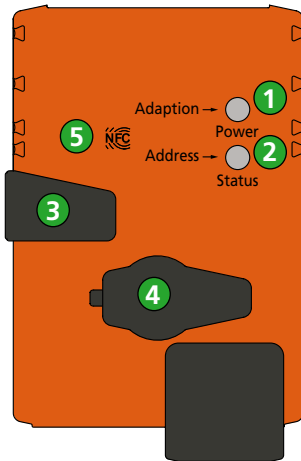
Abb. 11. Belimo-Stellantrieb.
