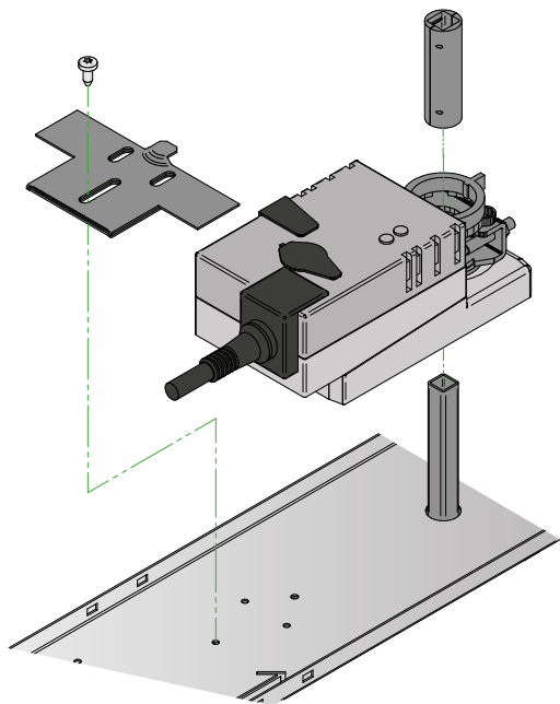
Abb. 17. Demontage des Klappenmotors.
