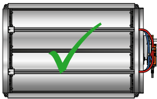
Abb. 6. Montage - Für rechteckige Kanäle wird die Klappe immer so montiert, dass der Regler/Stellantrieb parallel zum Kanal montiert wird.
