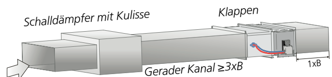
Abb. 8. Anforderungen an gerade Strecken 3 x B bei Schalldämpfern mit Kulisse. Gilt sowohl für Zu- als auch Abluft.
