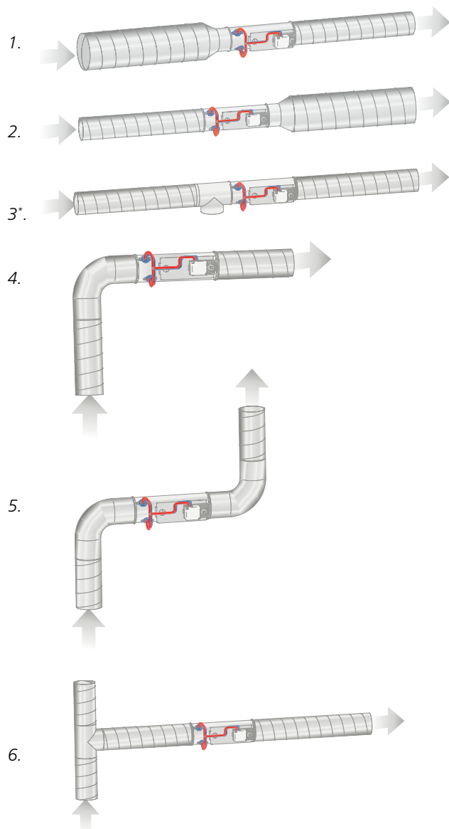
Abb. 5. Anforderungen an gerade Strecken in runden Kanälen, Anzahl Ø vor dem Produkt: Bilder 1–5 erfordern keine gerade Strecke (Bild 3* zeigt ein T-Stück mit Reinigungsdeckel). Bild 6 erfordert eine gerade Strecke vor der Klappe entsprechend 4 x Kanaldurchmesser.
