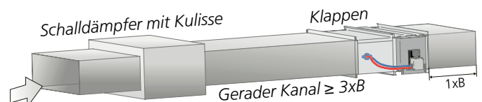
Abb. 11. Anforderungen an gerade Strecken 3 \times B bei Schalldämpfern mit Kulissee. Gilt sowohl für Zu- als auch Abluft.
