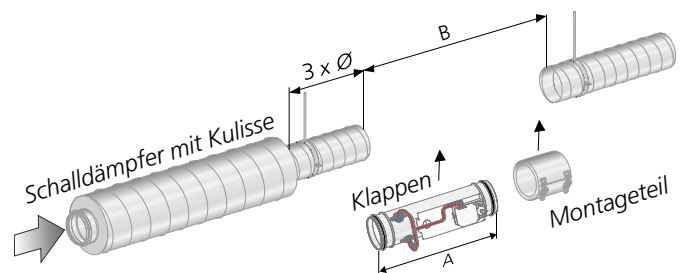
Abb. 6. Anforderung an gerade Strecken, 3 x Ø bei Schalldämpfer mit Kulissen oder Mittelkörper.
