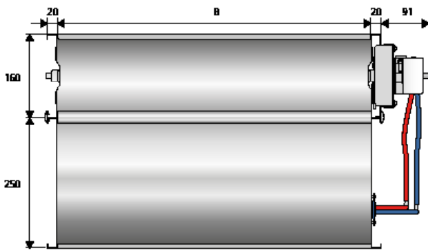
Abb. 8. Abmessungen (mm), REACT V SKNX rechteckig.
