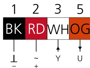
Abb. 2. Anschluss.
