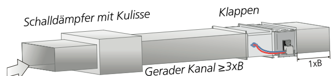
Abb. 10. Anforderungen an gerade Strecken 3 x B bei Schalldämpfern mit Kulissee. Gilt sowohl für Zu- als auch Abluft.
