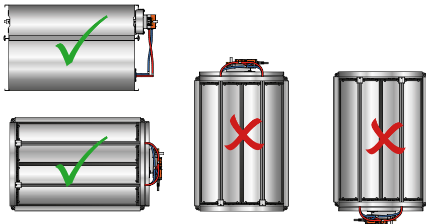
Abb 8. Montage - Für rechteckige Kanäle wird die Klappe immer so montiert, dass der Regler/Stellantrieb parallel zum Kanal montiert wird.
