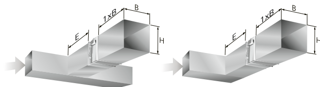
Abb. 9. Anforderung an gerade Strecken in rechteckigen Kanälen.
