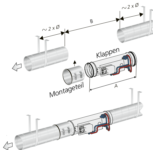
Abb. 6. Installation im Kanalsystem. Die Kanäle müssen in der Gebäudekonstruktion auf allen Seiten des Produkts fixiert werden.
