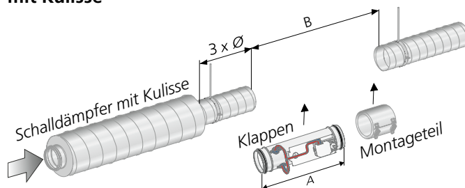
Abb. 5. Anforderung an gerade Strecken, 3 x \emptyset bei Schalldämpfer mit Kulissen oder Mittelkörper.
