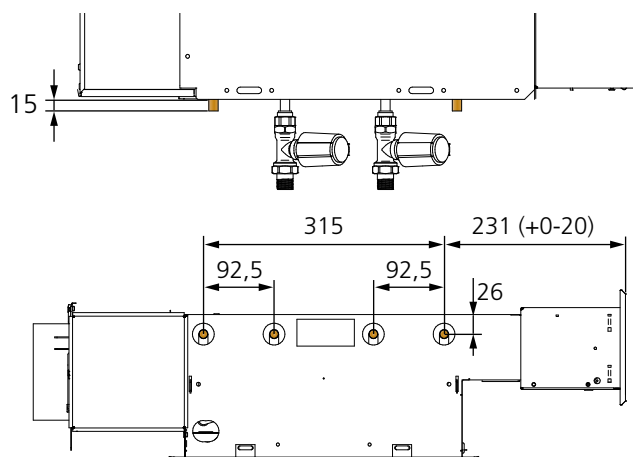
Figur 15. Mått, upphängning.
