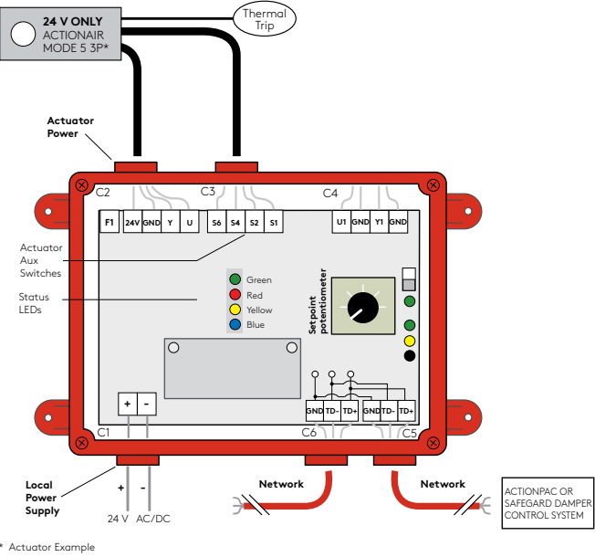
Figure 10. 3P-SFDI-M/FT 24 V Auto Mode.
