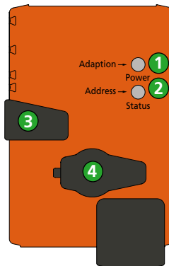
Figure 1. Régulateur REACT V BMB. 1. Bouton-poussoir et voyant LED vert 2. Bouton-poussoir et voyant LED jaune 3. Bouton de libération des engrenages 4. Port service
