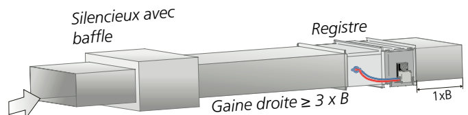
Figure 10. Exigences relatives à la section de gaine droite 3 x B en cas de silencieux avec baffle. S'applique à l'alimentation et à l'extraction d'air.
