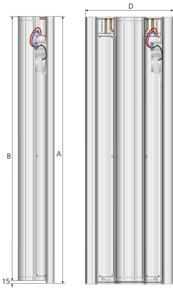
Figur 13. Måttskiss - fullstorlek.
