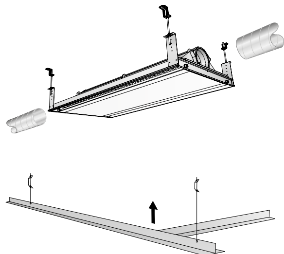
Figur 18. Upphängningsvariant med montageband respektive gångstång.
