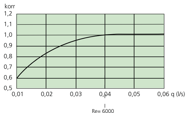
Diagram 2. Vattenflöde – kapacitetskorrektion, värme
