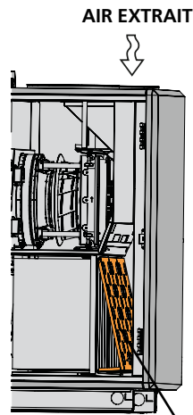
Plaque d'équilibrage Accrocher les plaques d'équilibrage sur le guide du filtre supérieur, puis enfoncer les plaques d'équilibrage vers le bas pour qu'elle se fixe dans le guide inférieur.
