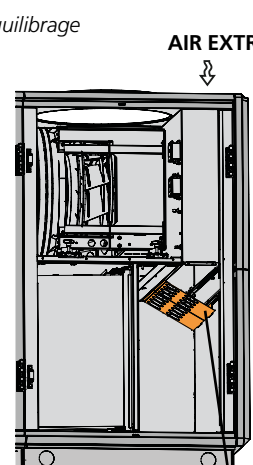
Plaque d'équilibrage Accrocher la plaque d'équilibrage dans l'encoche du côté du filtre. Soulever la plaque d'équilibrage vers le caisson de la CTA et l'accrocher dans l'encoche.
