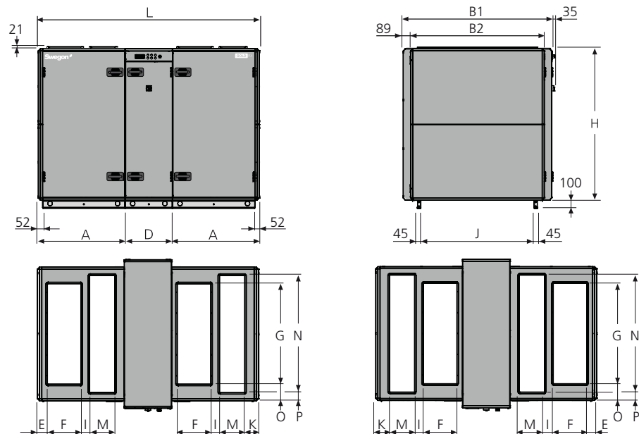
Vue du dessus. Montre les raccords de gaine de la centrale de traitement d'air pour le ventilateur d'air soufflé en haut à droite et en bas à gauche
