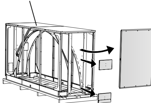
Bovenste behuizingssectie
