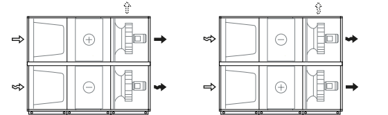
Ventilatoropstelling 5, toevoerlucht hoger
