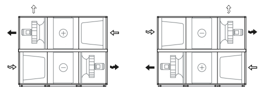
Ventilatoropstelling 1
