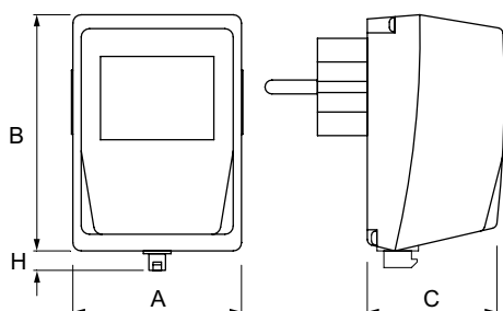
Figur 1. POWER A 20 VA.
