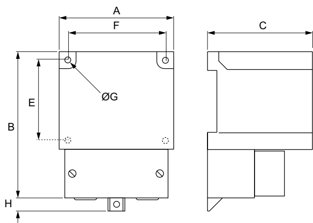
Figur 2. POWER A 60 VA (3 st skruvhål) samt POWER A 150 VA (4 st skruvhål).
