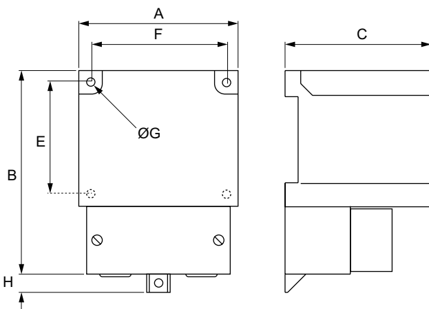
Kuva 2. POWER A 60VA (3 ruuvireikää) sekä POWER A 150VA (4 ruuvireikää).
