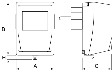
Kuva 1. POWER A 20VA.
