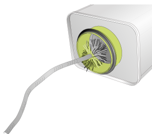
Figur 2. Rengöring med plastviska
