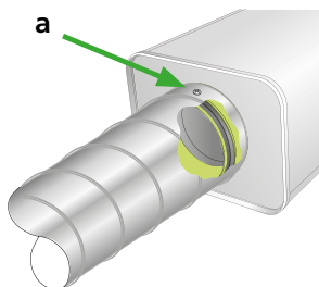
Figur 1. Fäst anslutningskanalen i den uppdragna plåtkanten som är fastgjuten inuti anslutningstosen med skruv eller popnit (a).
