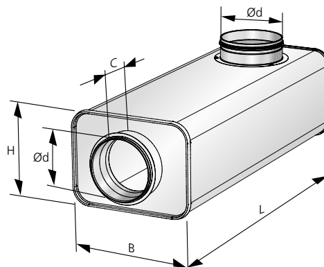
Figur 3. CLV – måttskiss
