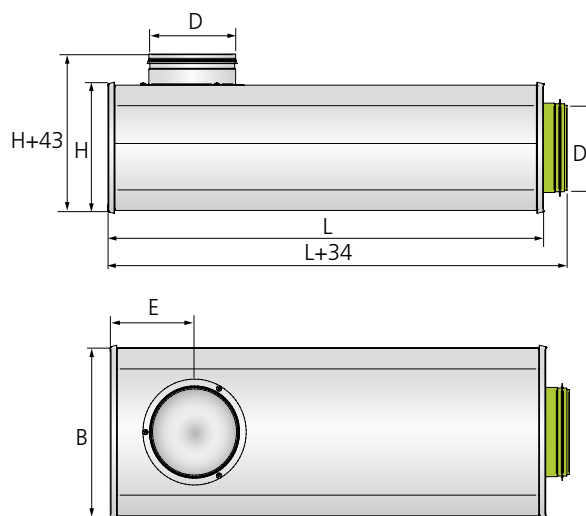
Figur 4. CLV – måttskiss från sidan
