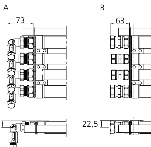
Figur 14. Anslutningsdetaljer. A = Röravslut, B = Rörinkoppling
