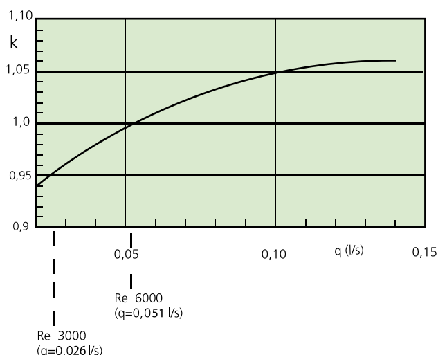
Diagram 3a. Vattenflöde-effektkorrektion
