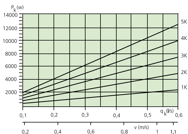
Diagram 2. Vattenflöde-kyleffekt, per gren.
