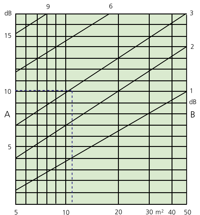
Käyrästä 6. Reduktiokerroin
