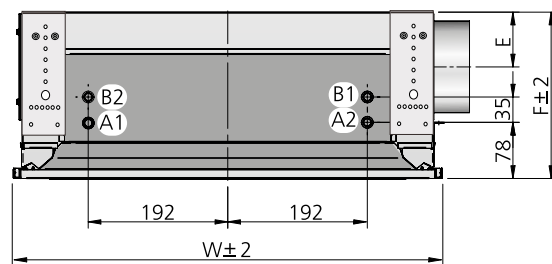
Figur 27. Parasol 1200, gavelvy och anslutningar
