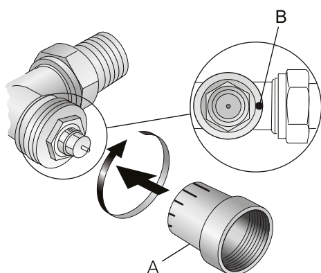
Figur 16. Injustering av k_v -värde
