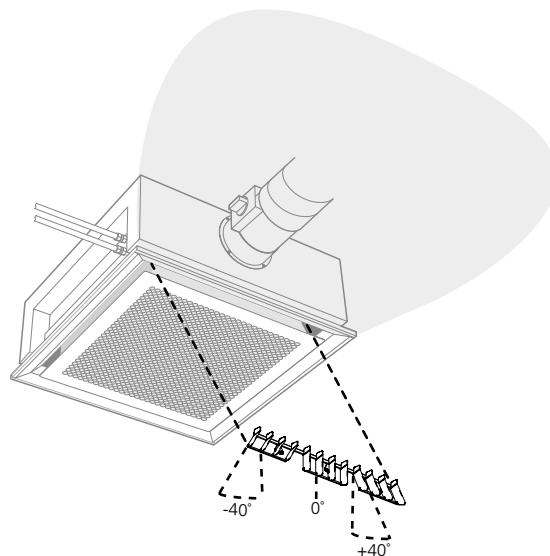
Figur 7. Inställningsmöjligheter ADC I , Fan-shape
