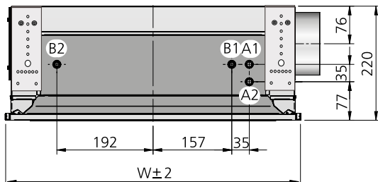
Figur 25. Parasol 600, gavelvy och anslutningar
