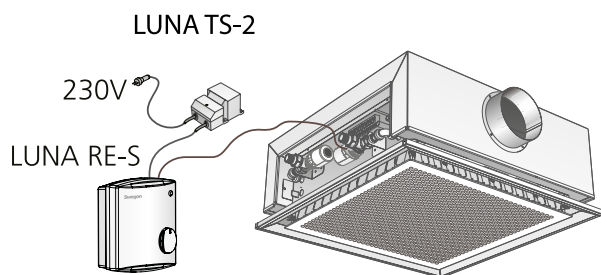
Figur 14. Typinstallation, vattenburen kyla och värme
