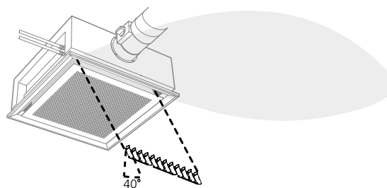
Figur 8. Inställningsmöjligheter ADC I , X-shape
