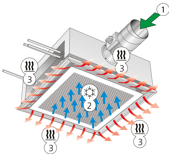
Figur 2. Variant B: Värme- och tilluftsfunktion (inkluderar även kylfunktion)
