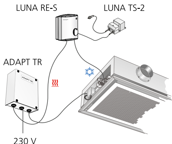
Figur 15. Typinstallation, vattenburen kyla samt elvärme
