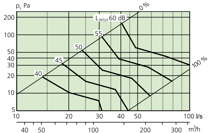
Diagram 7. Injusteringsområde, spjäll, CRPc 9-125
