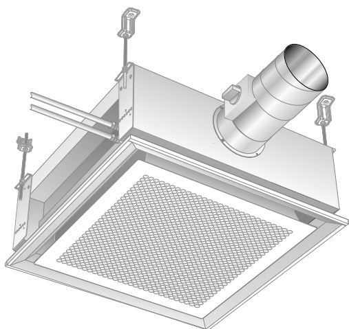
Figur 17. Upphängning enmodulsenhet
