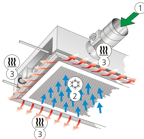
Figur 4. Variant X: Tilluft- och värmefunktion med elstavar (inkluderar även kylfunktion)
