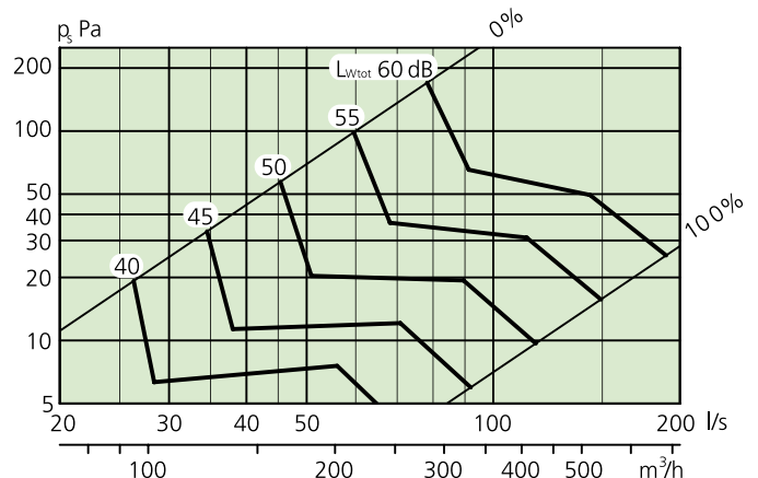
Diagram 8. Injusteringsområde, spjäll, CRPc 9-160
